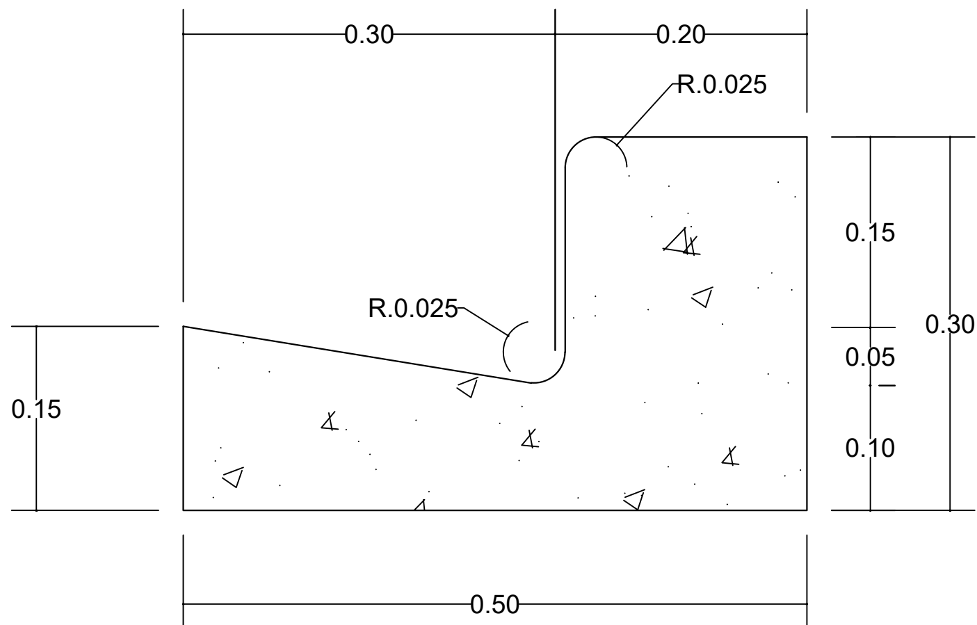
SECCION TRANSVERSAL CONTENES DE 0.50 L
